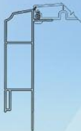
Moulure extérieure à déclin 4 po
